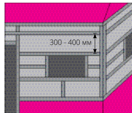
рис. 26 Горизонтальная обрешетка
